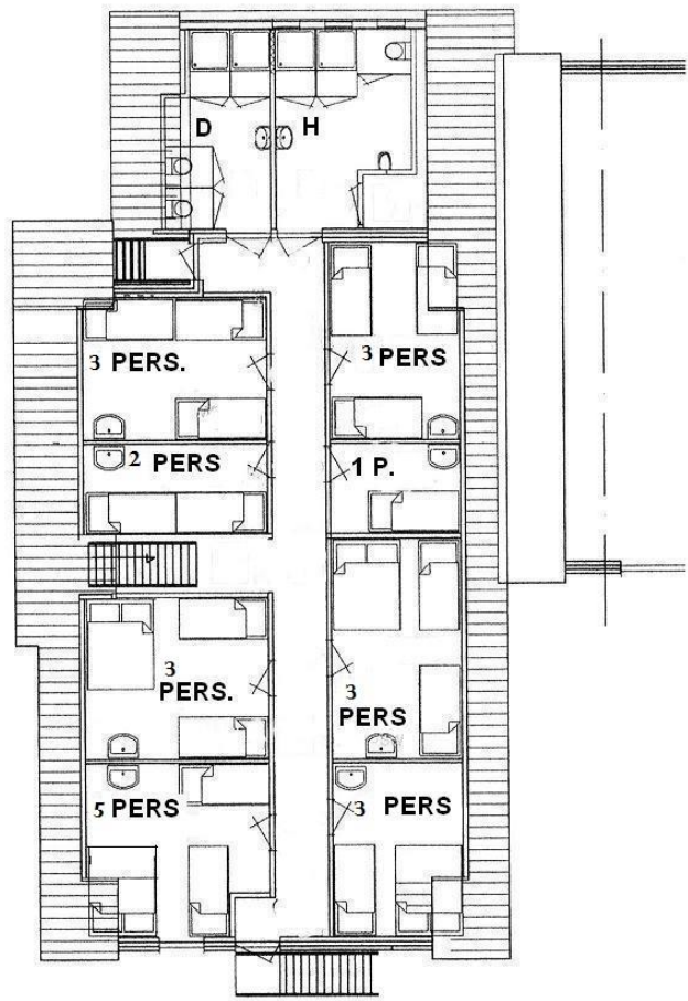
VERDIEPING
